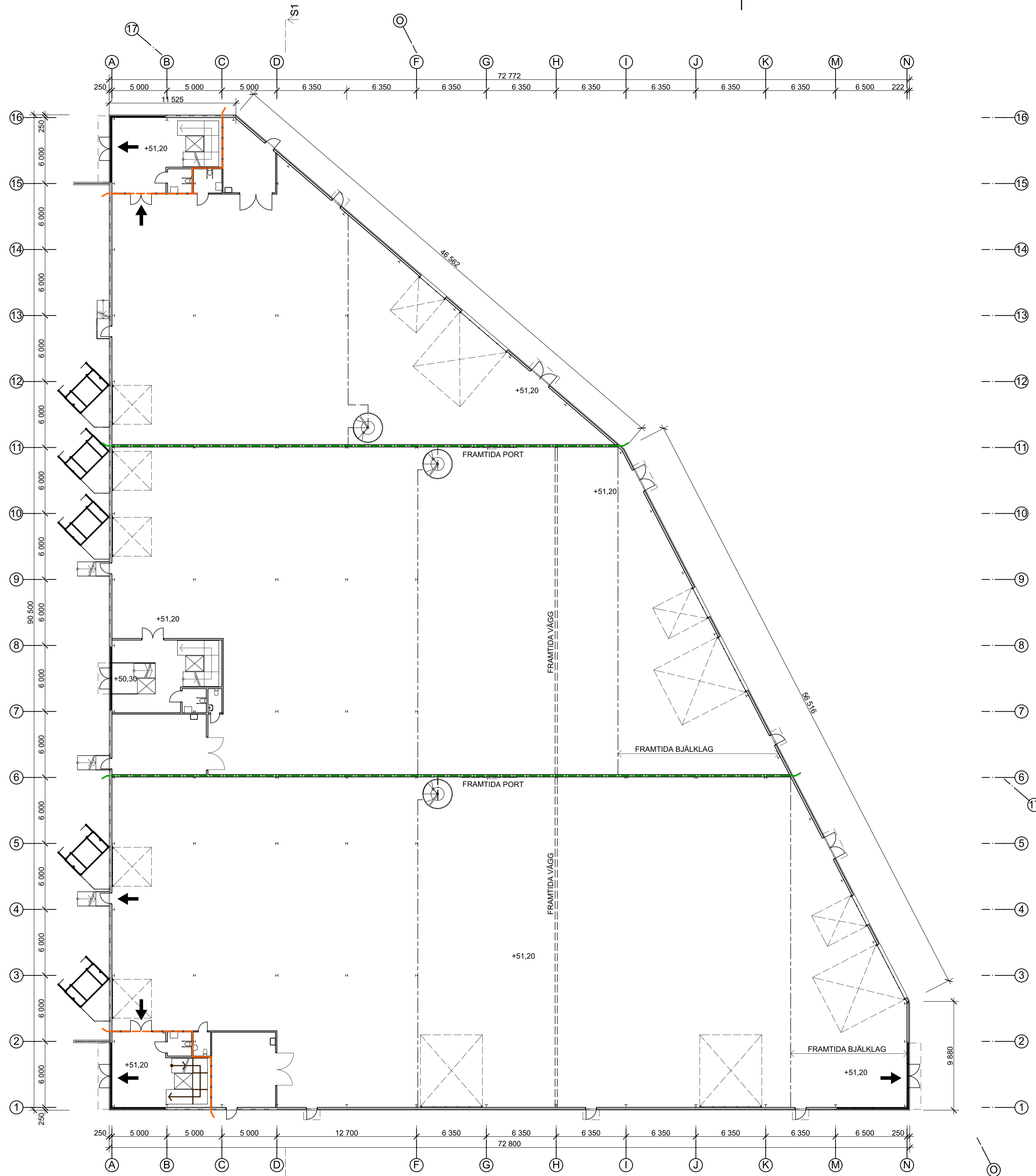
VÅNING 1 - BOTTENPLAN 1:200
